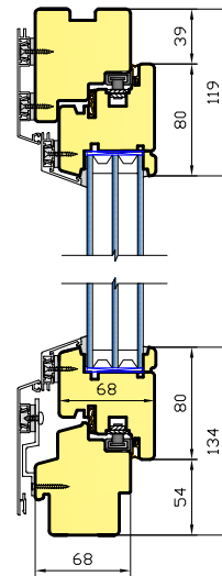
Lõige B-B 1:1
