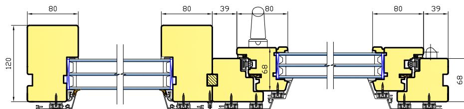
Lõige C-C 1:1
