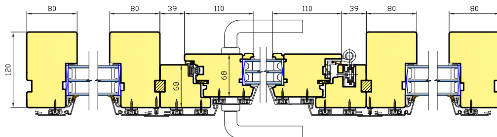
Lõige C-C 1:1
