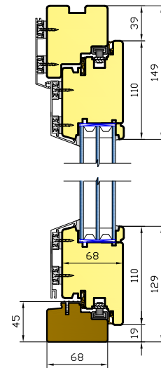
Lõige B-B 1:1
